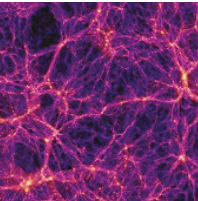
Datasimulering av det kosmiske nettverket, der hver prikk er en galakse. Foto: Volker Springel / Max Planck Institute For Astrophysics
